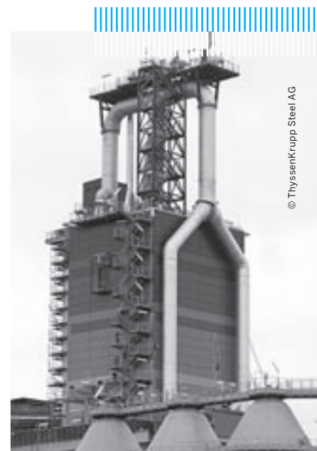
Der neue Hochofen 8 der ThyssenKrupp Steel AG steht für die Zukunft des Stahlstandortes Duisburg.
